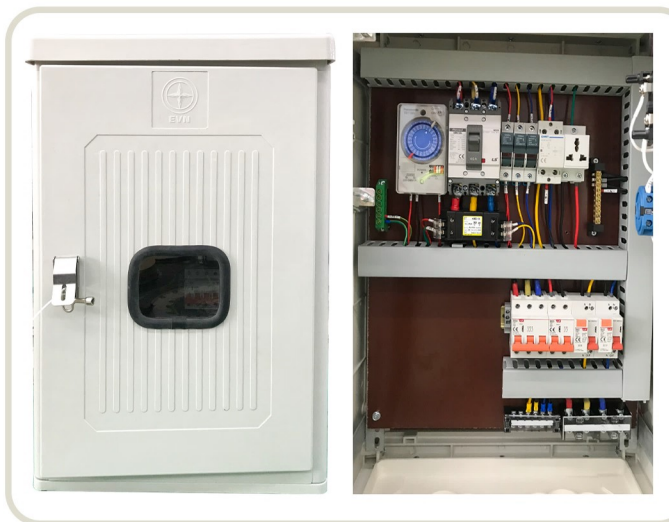
Tủ chiếu sáng
