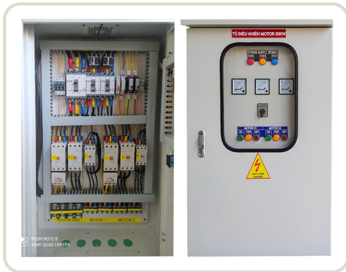
Tủ điều khiển motor 30KW
