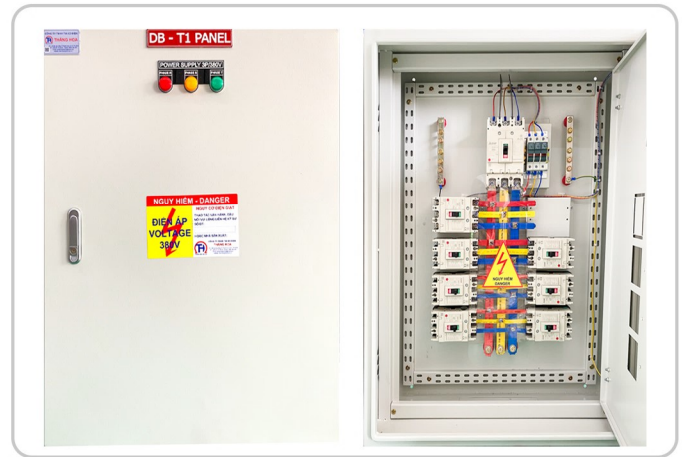
Tủ DB 250A
