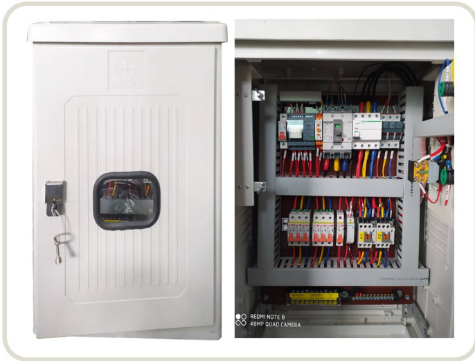
Tủ chiếu sáng
