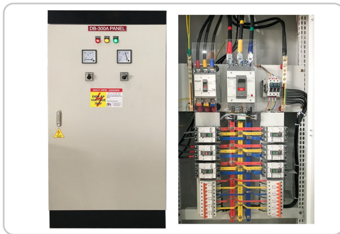
Tủ DB 300A
