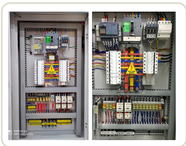
Tủ điều khiển bơm nước
