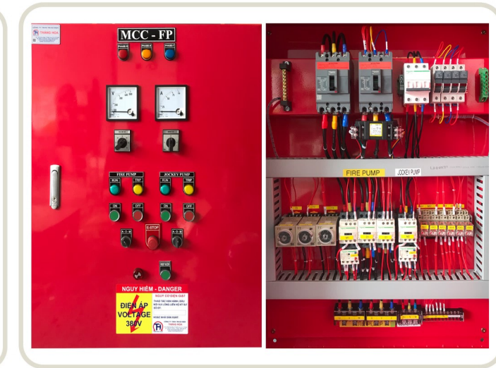
Tủ bơm PCCC
