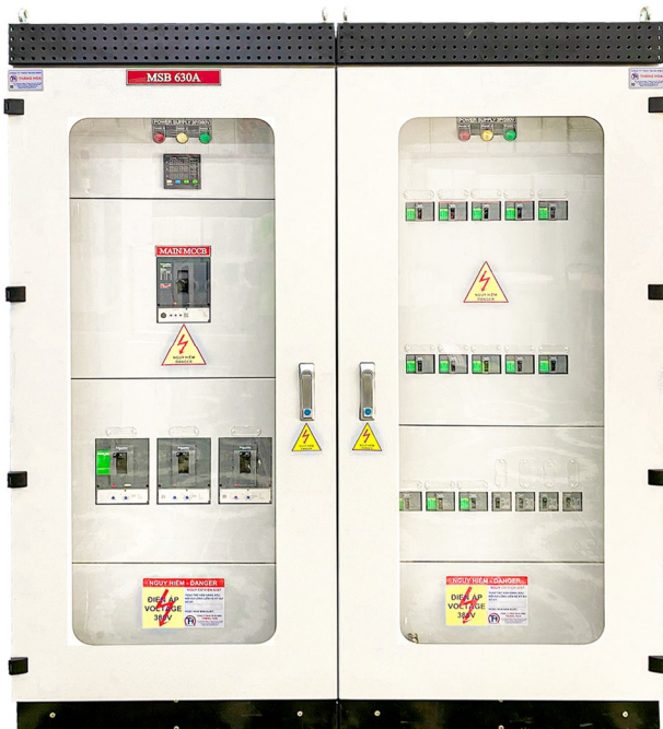
Tủ MSB 630A
