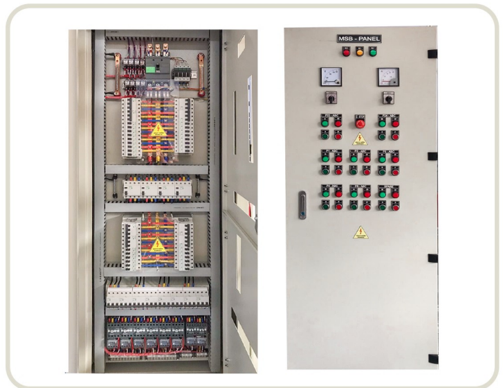
Tủ MSB và điều khiển quạt gió
